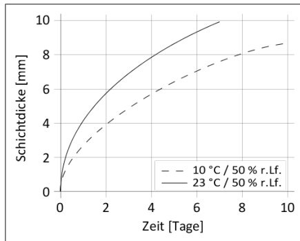
Diagramm 1: Durchhärtegeschwindigkeit Sikaflex®-221
